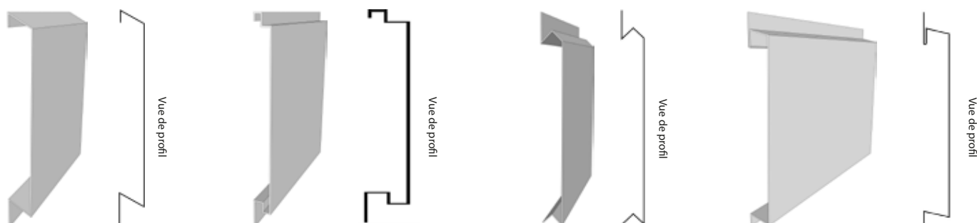
CL11 - Méline C
