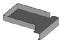
BA11 22 Bavette 3 plis avec relevés latéraux et moustaches
